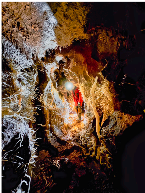
Geologiaren eszentrikotasuna
